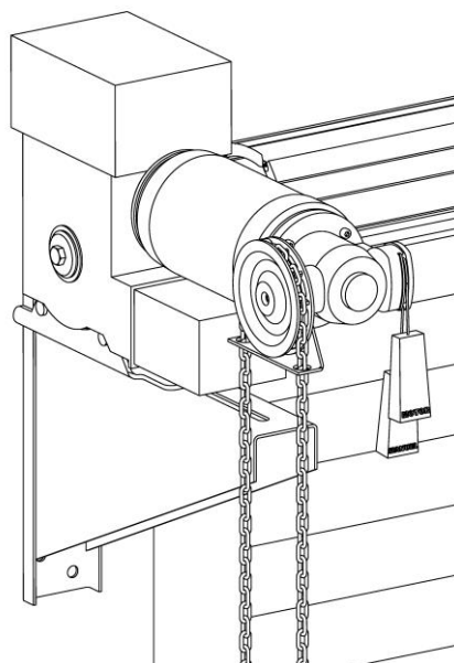
Rys.5. Napęd awaryjny łańcuchowy
