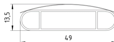
Widok belki dolnej z lamelą
