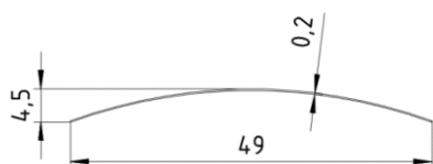
Widok lameli
