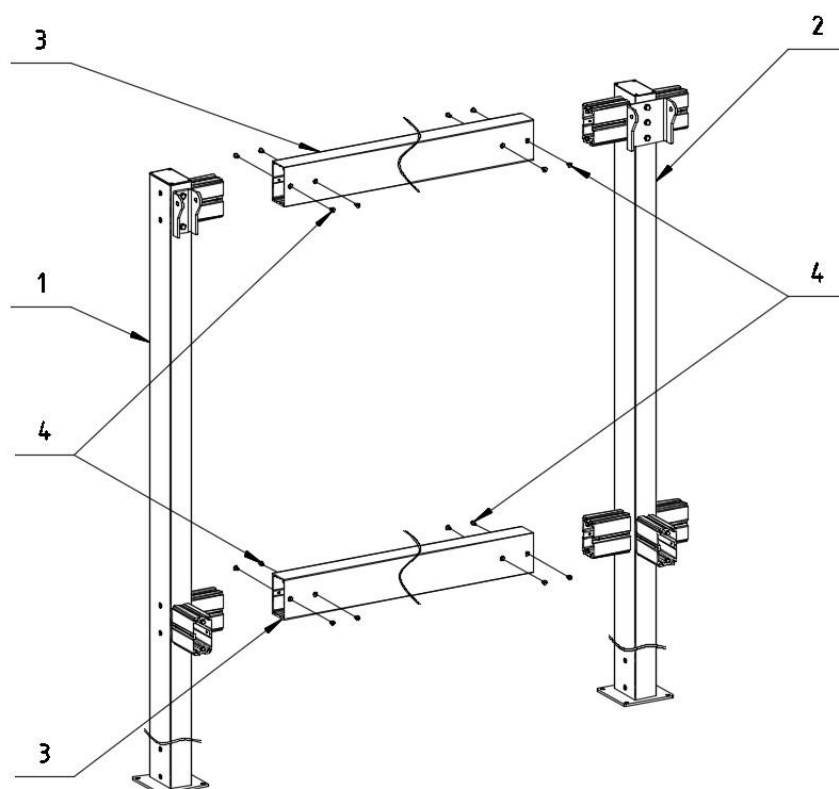
Rys. 24. Sposób montażu Belki tylnej pierwszego modułu. 1 - Słup wysoki (lewy / prawy), 2 - Słup wysoki (pośrodkni), 3 – Belka tylna, 4 - Śruba M8x16.
