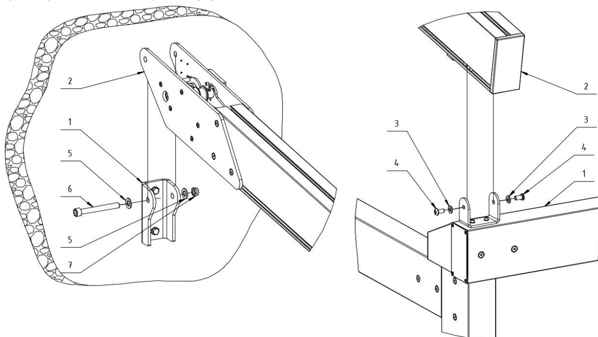
Rys. 42. Sposób montażu Belki prowadzącej: 1 - Konstrukcja nośna, 2 - Belka prowadząca, 3 - Podkładka \varnothing 10,5 , 4 - Śruba M10x20, 5 - Podkładka \varnothing 15 , 6 - Śruba M14x120 / M14x220, 7 - Nakrętka M14.
