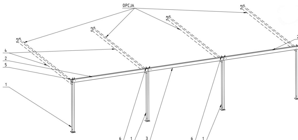
Rys. 34. Konstrukcja nośna wersja przyścienna modułowa: 1 - Słup niski 2 - Belka przednia (prawa, lewa), 3 - Belka przednia (pośrodkowa) 4 - Belka boczna, 5 – Rynna, 6 - Uchwyt belki prowadzącej modułowej.
