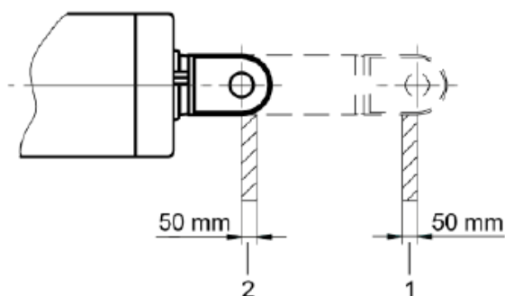
Rysunek 34 Dopuszczalna redukcja skoku silnika
