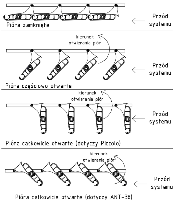
Rys. 3. Standardowe ustawienie kierunku otwierania piór w Pergoli SB500.
