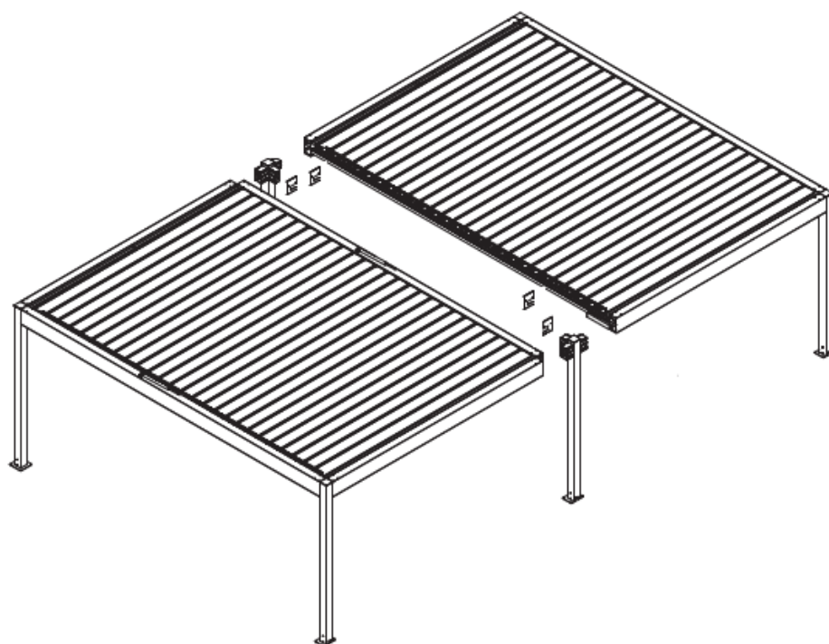
Rys. 4b. Widok montażu modułów Pergoli SB500.
