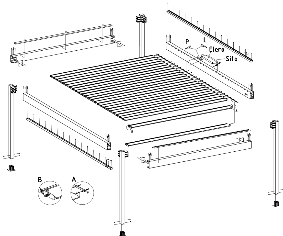
Rys. 4a. Widok montażu elementów Pergoli SB500 wolnostojącej.
