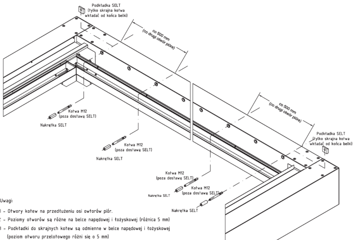
Rysunek 38 - Montaż przyścienny do belki wzdłużnej.
