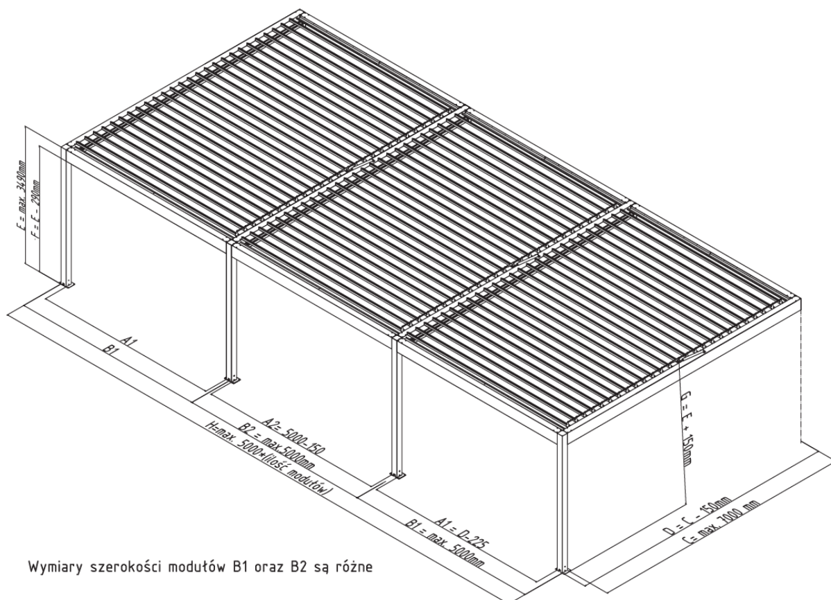
Rys. 2a. Pergola SB500 modułowa przyścienna poprzeczna (mocowanie przyścienne przelotowe przez belkę)
