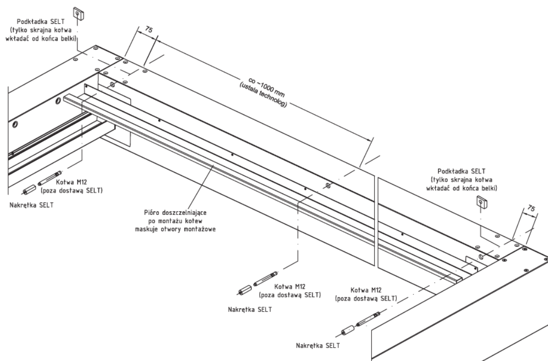
Rysunek 37 - Montaż przyścienny do belki tylnej/przedniej.
