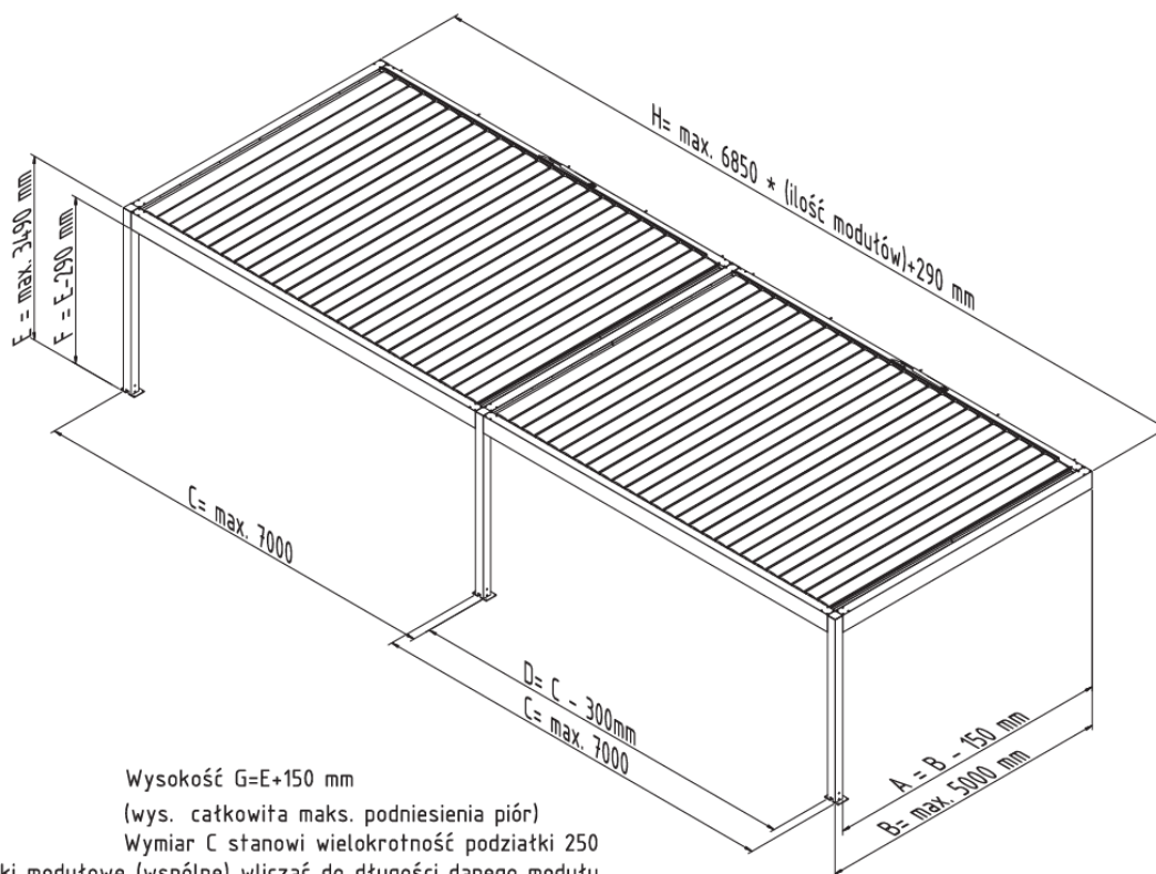
Rys. 2b. Pergola SB500 modułowa przyścienna podłużna (mocowanie przyścienne przelotowe przez belkę)
